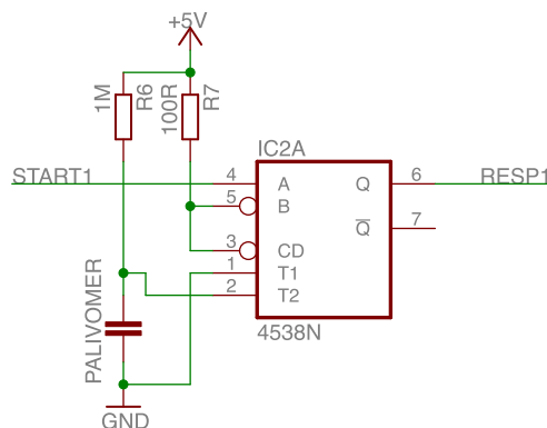
Obrázek 6: Zapojení palivoměru do obvodu. Integrovaný obvod 4538 po spuštění vygeneruje impuls dlouhý podle kapacity připojeného kondenzátoru.
